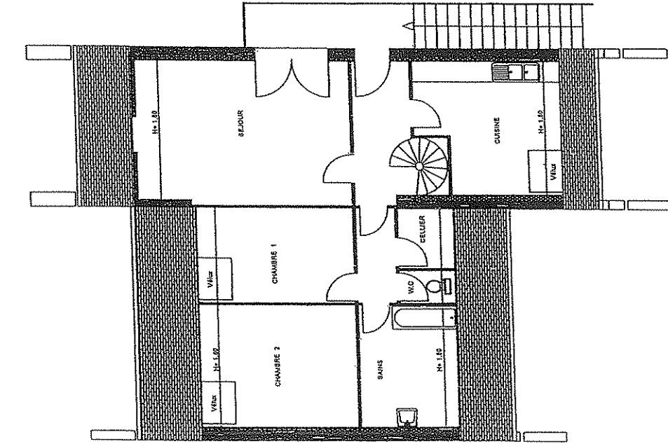
1° Partie du F 4 situé au 1° Etage du bâtiment
